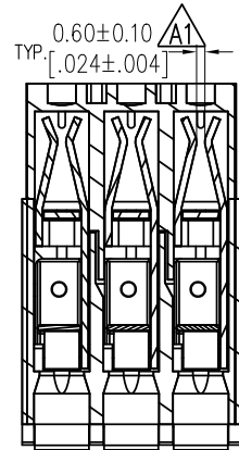
SEC A-A
